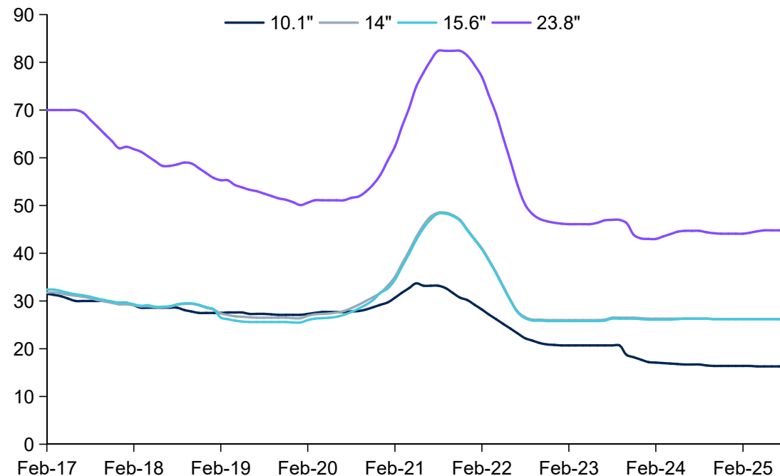
图：10.1、14、15.6、23.8英寸LCD IT面板价格走势（单位：美元）
