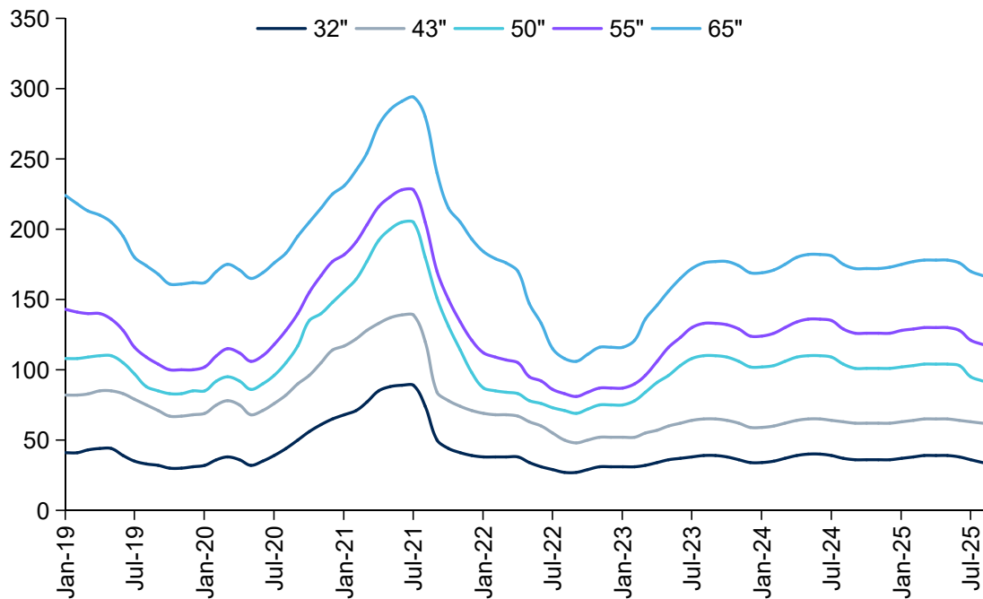
图：32、43、50、55、65英寸LCD TV面板价格走势（单位：美元）
