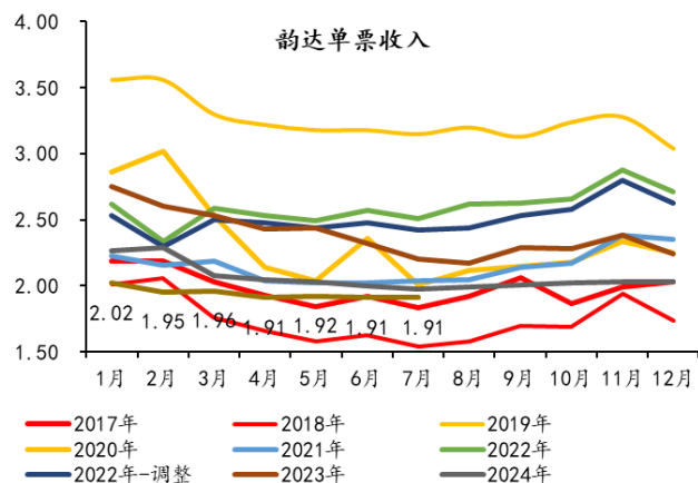
图6：韵达单票收入（元）
