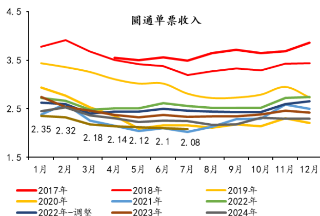
图5：圆通单票收入（元）
