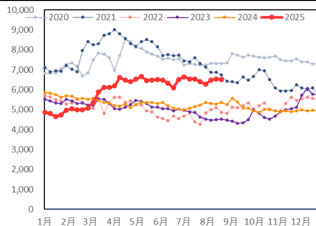
图 46: 原油、无规聚丙烯价差 (元/吨, 元/吨)
