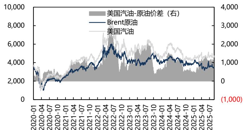
原油、美国汽油价格及价差（元/吨，元/吨）
