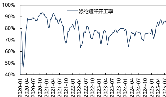
2020-2025年涤纶短纤开工率 (%)
