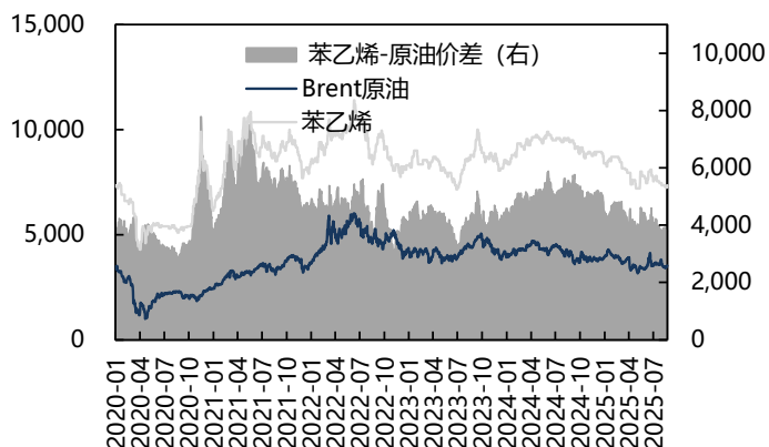
原油、苯乙烯价格及价差 (元/吨, 元/吨)
