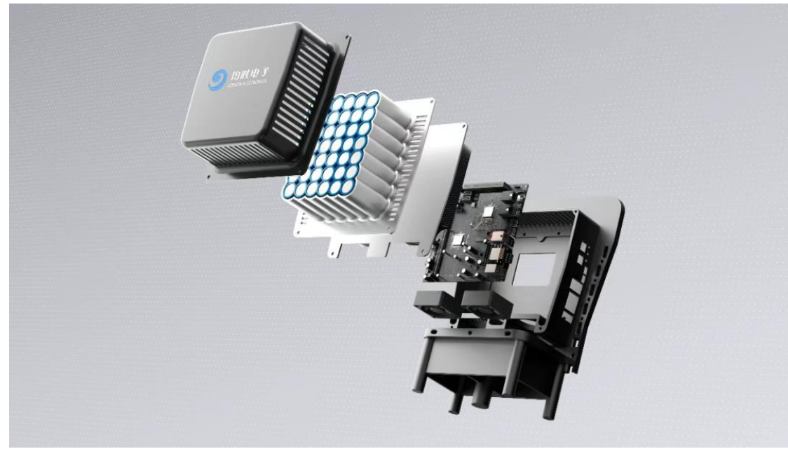
图表：均胜电子双足人形机器人胸腔总成方案
