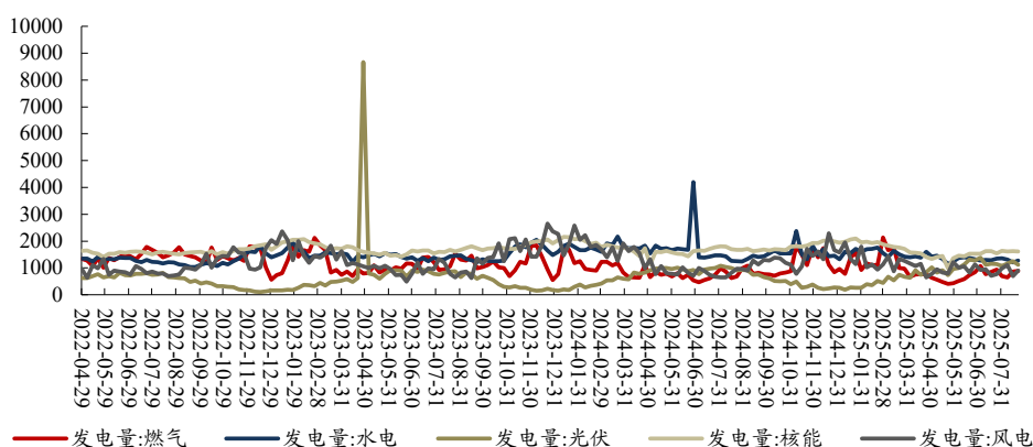
图7：最近一年欧洲发电结构（GWh/日，周度数据，截至 2025/8/22）
