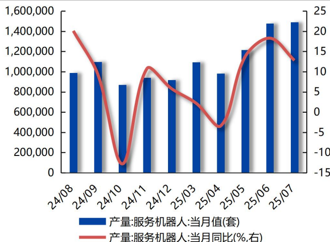
图表 20：中国服务机器人 7 月产量同比+12.8%
