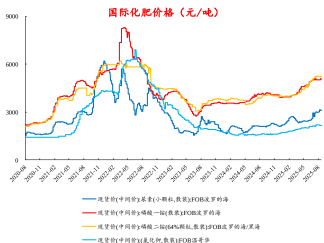
图18：本周国际尿素价格下跌
