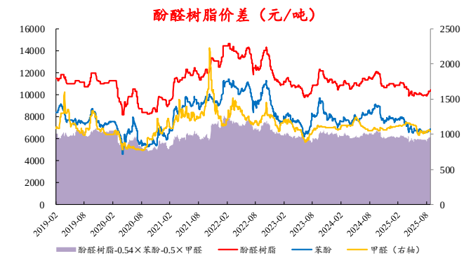
图32：本周酚醛树脂价差小幅扩大
