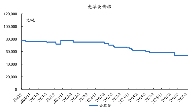
图57：本周麦草畏价格稳定
