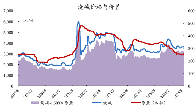
图46：本周烧碱价差扩大
