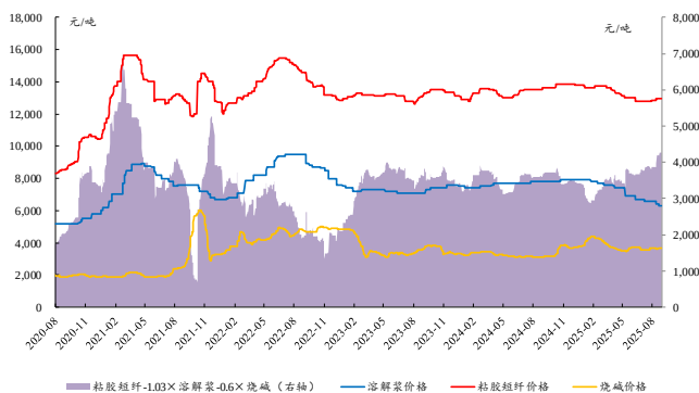
图9：本周粘胶短纤价差缩小
