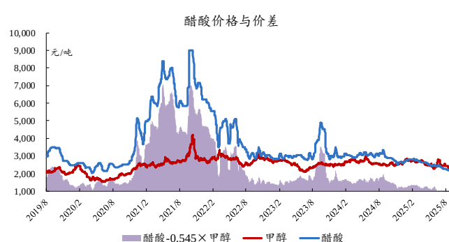
图42：本周醋酸价差缩小
