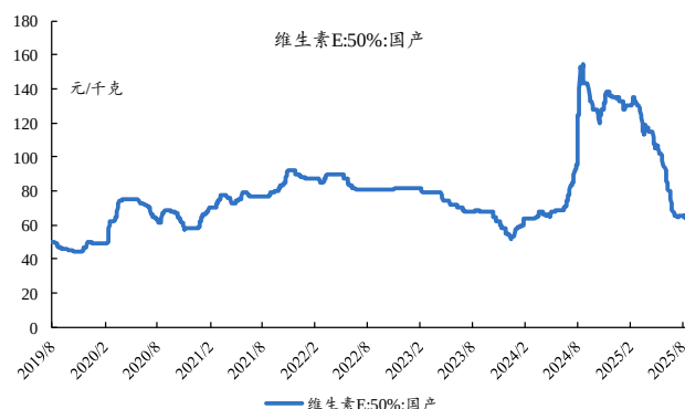
图60：本周维生素E价格下滑
