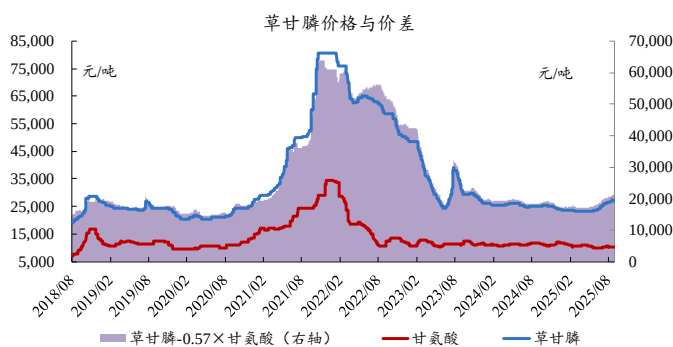
图53: 本周草甘膦价差扩大
