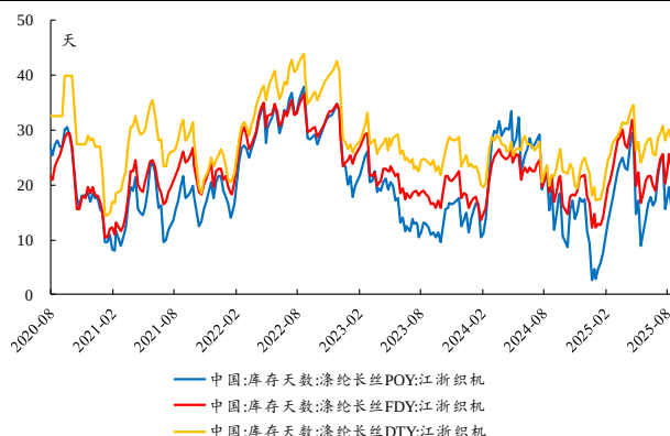
图8：本周涤纶长丝 POY 库存天数上升
