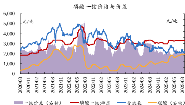
图51: 本周磷酸一铵价差扩大
