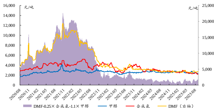
图41：本周DMF价差扩大
