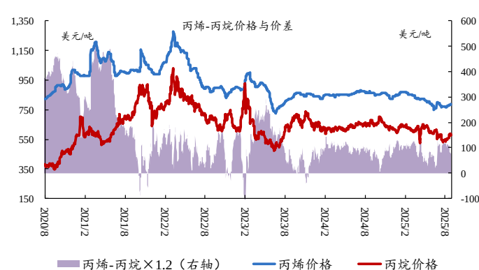
图25：本周丙烯-丙烷价差扩大
