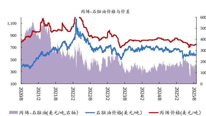
图26：本周丙烯-石脑油价差收窄
