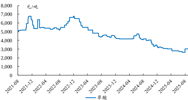
图48：本周草酸价格基本稳定
