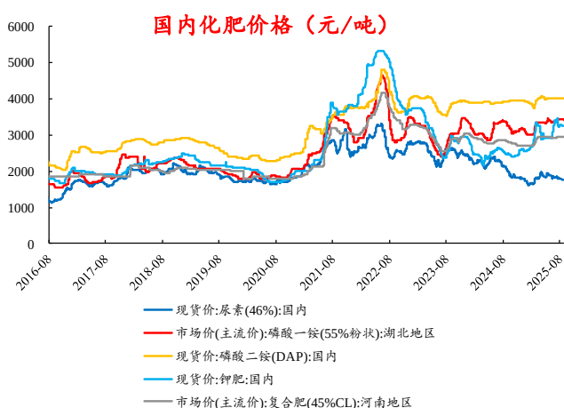
图17：本周国内尿素价格下跌
