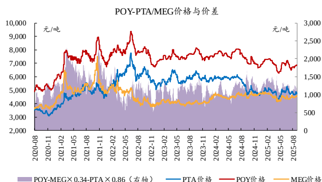
图7：本周涤纶长丝 POY 价差扩大
