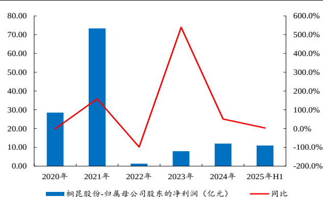
图6：2025H1 桐昆股份归母净利润同比+2.93%
