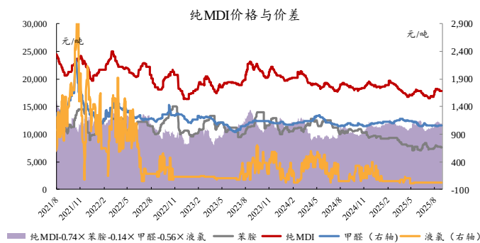
图19：本周纯 MDI 价差收窄
