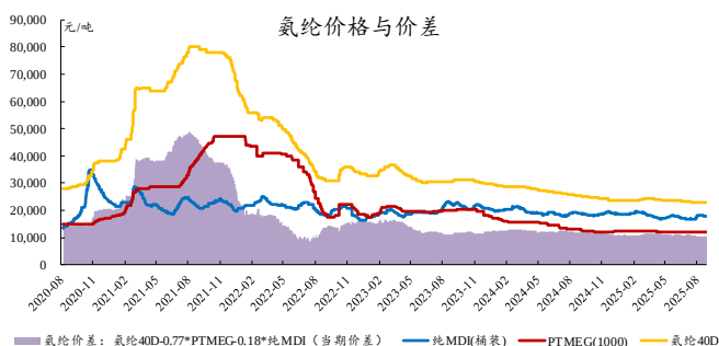
图13：本周氨纶价差基本维持稳定
