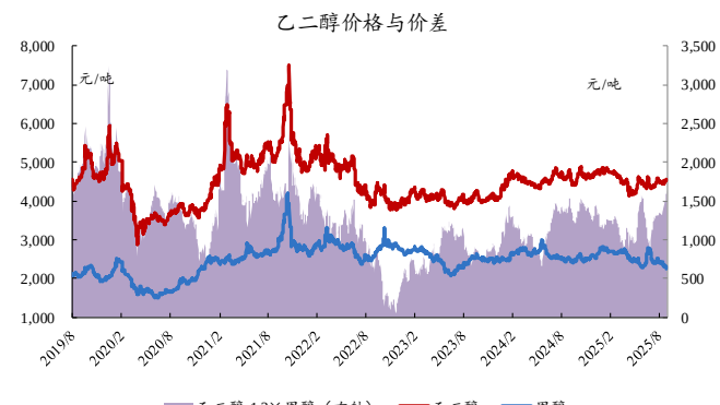
图44：本周乙二醇价差扩大
