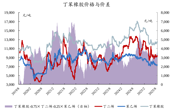
图30：本周丁苯橡胶价差扩大
