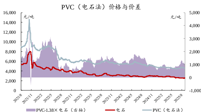
图45：本周 PVC（电石法）价差收窄
