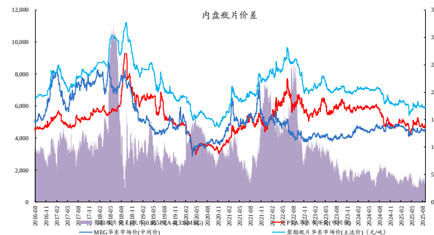
图31：本周瓶片价差收窄
