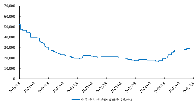
图58：本周百菌清价格稳定
