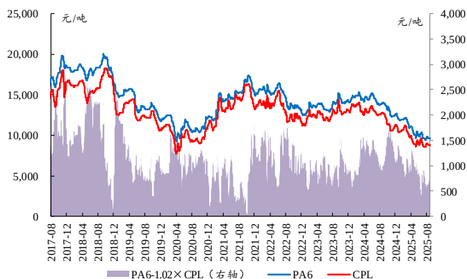
图37：本周 PA6 价差扩大
