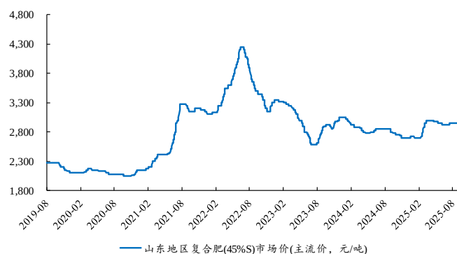
图49：本周复合肥价格维持稳定
