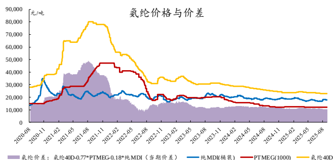
图33：本周氨纶价差不变
