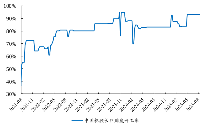
图12：本周粘胶长丝行业开工率持稳运行
