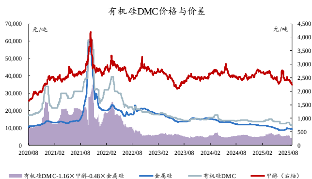
图39：本周有机硅DMC价差扩大
