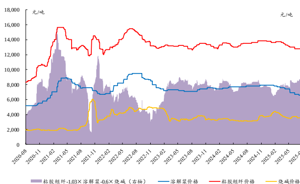
图35：本周粘胶短纤价差小幅缩小
