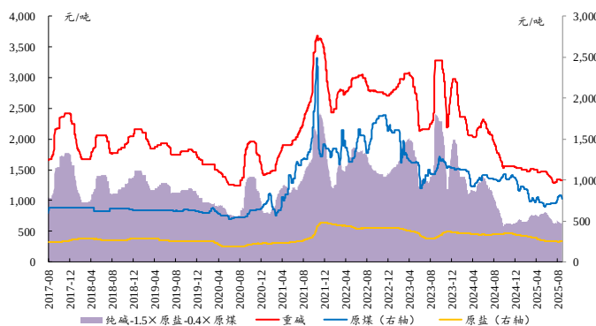
图47：本周纯碱价差小幅扩大
