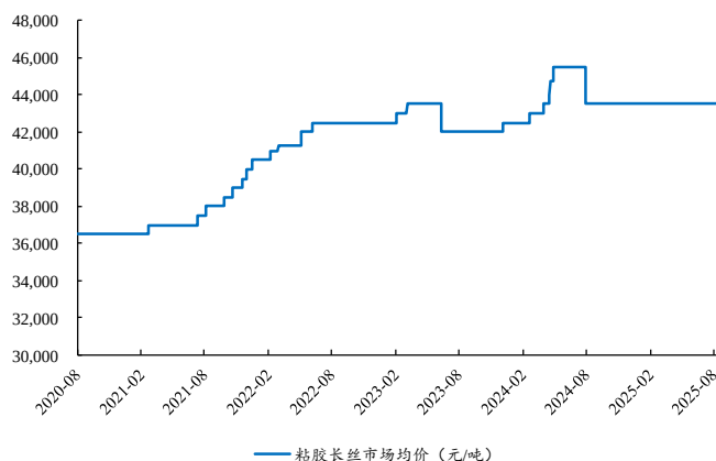
图36：本周粘胶长丝市场均价保持稳定
