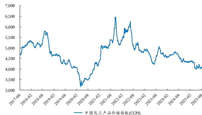
图2：8 月 29 日 CCPI 报 4009 点，较上周五下跌 0.55%
