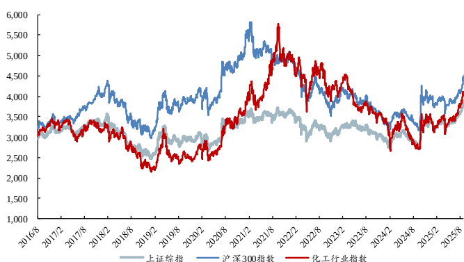
图1：本周化工行业指数跑输沪深 300 指数 1.6%
