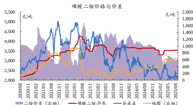
图52: 本周磷酸二铵价差扩大
