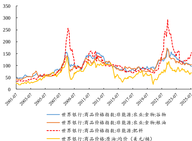
图15：2025年7月，肥料价格指数环比上升
