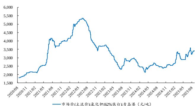
图50：本周国内氯化钾价格基本稳定
