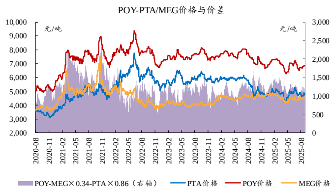
图24：本周POY-PTA/MEG 价差扩大
