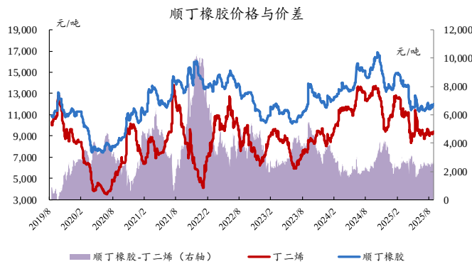
图29：本周顺丁橡胶价差扩大
