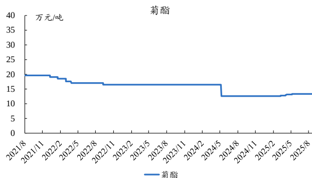
图56: 本周菊酯价格稳定
