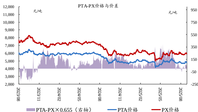
图23：本周PTA-PX 价差收窄
