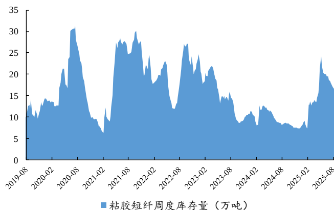
图10：本周粘胶短纤库存小幅降低
