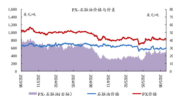
图22：本周PX-石脑油价差小幅扩大
