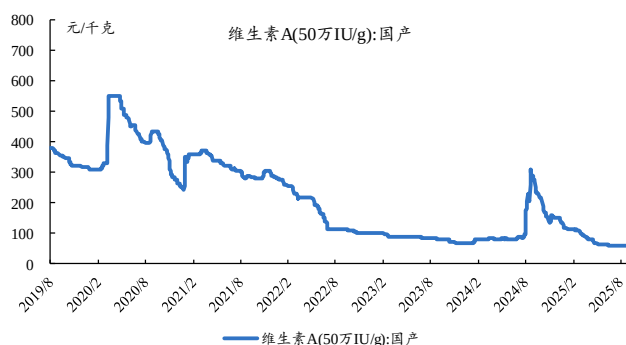
图59：本周维生素A价格基本稳定
