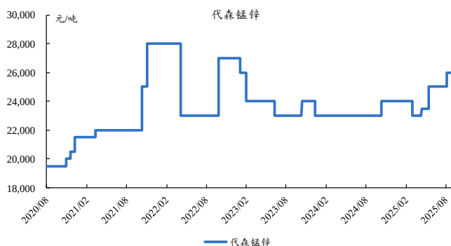
图55: 本周代森锰锌价格稳定
