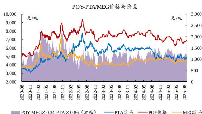
图34：本周 POY-PTA/MEG 价差扩大
