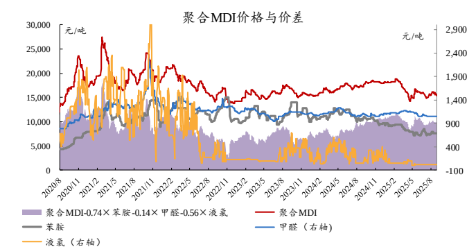
图20：本周聚合 MDI 价差收窄
