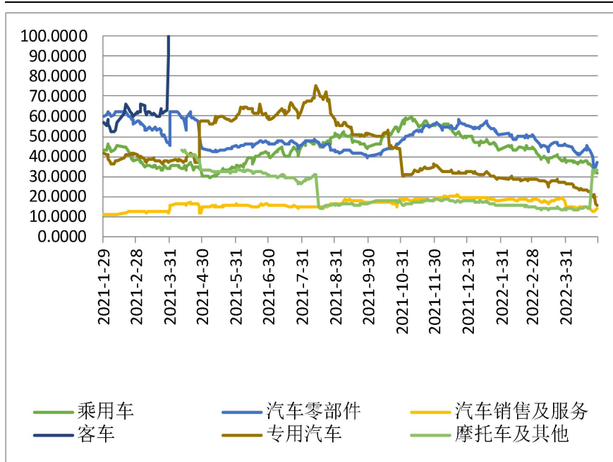
图 5：部分细分行业 PE(TTM)变化
