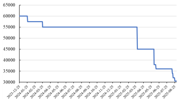
图表16：普鲁士蓝类化合物材料价格，元/吨
