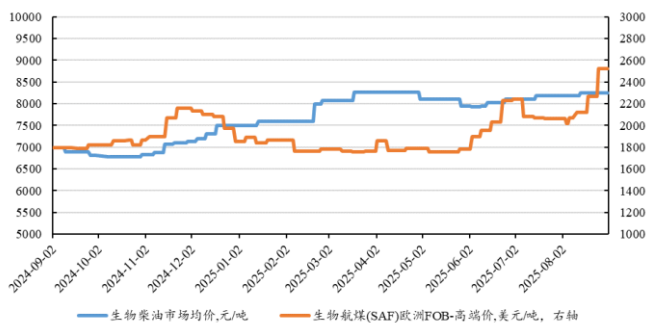
图表23：生物柴油及 SAF 价格
