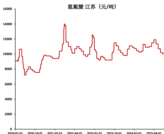
图 7：氢氟酸价格走势
