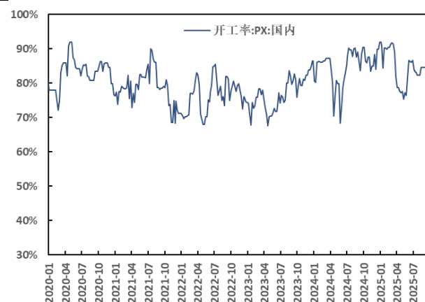
图 59: PX 开工率 (%)
