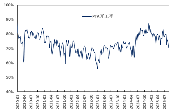
图 67: PTA 开工率 (%)
