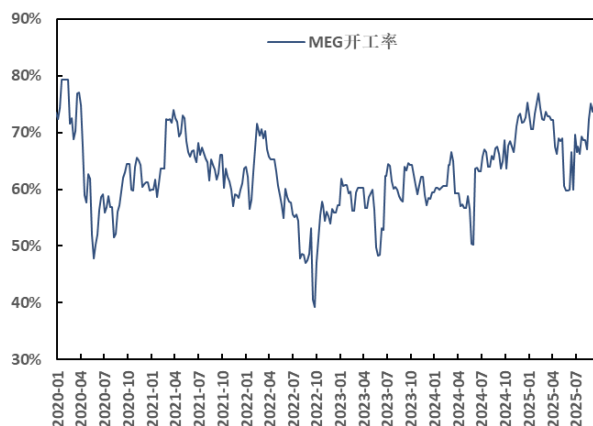
图 61: MEG 开工率 (%)
