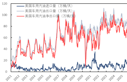
图 64：美国车用汽油进出口情况（万桶/天）
