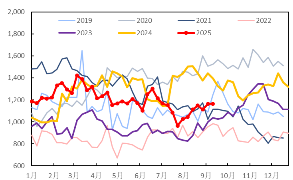
图 81: 新加坡柴油库存 (万桶)
