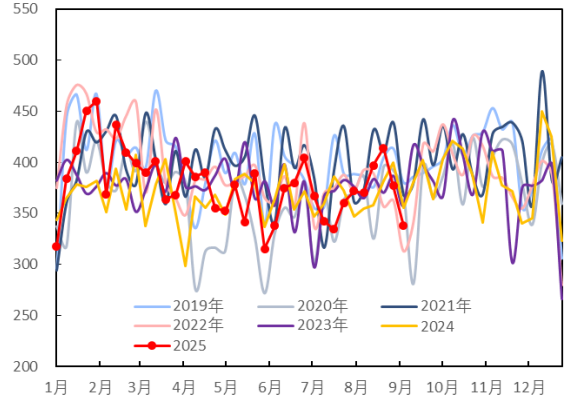
图 61：美国柴油消费量（万桶/天）
