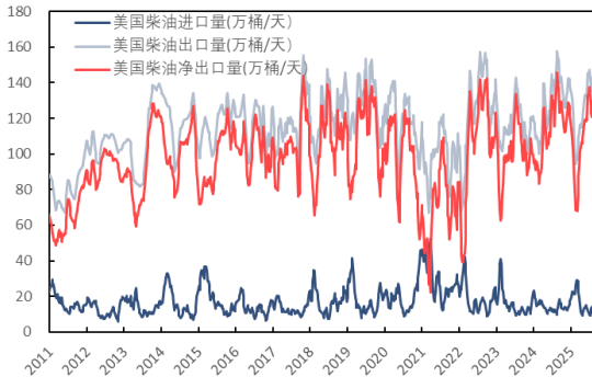
图 66：美国柴油进出口情况（万桶/天）
