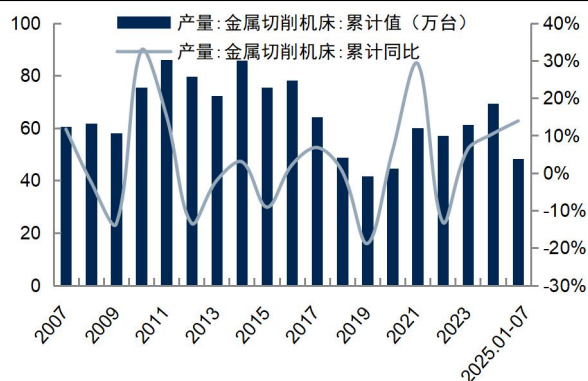
图19：2025 年 1–7 月金属切削机床产量累计同比增长 13.90%
