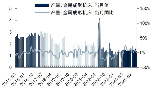
图20：2025 年 7 月金属成形机床产量同比增长 0.00%
