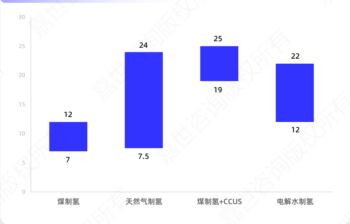
0.2元/kwh制氢成本对比
