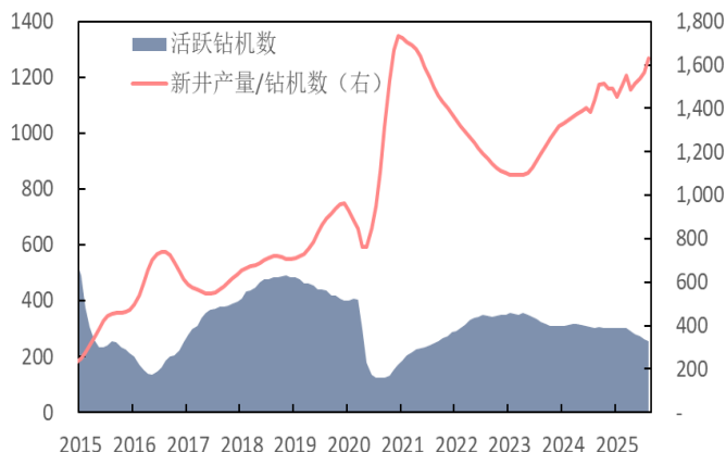
图 55: 美国 Permian 产区钻机数量和单个钻机对应的新井原油产量 (台, 桶/日)
