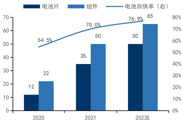
图5：电池组件年底产能（GW）
