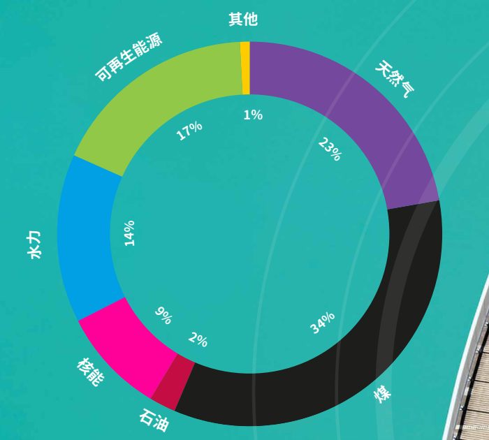
2024年，低碳和零碳能源的发电量超过总发电量的40%
