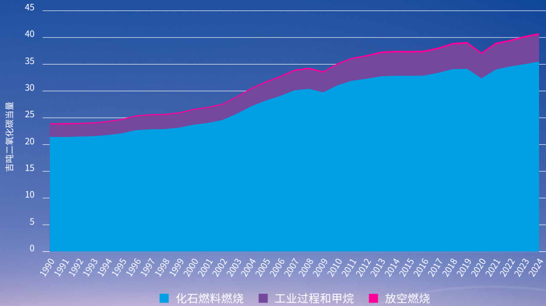
自新冠疫情以来，全球排放量年均增长2.3%
