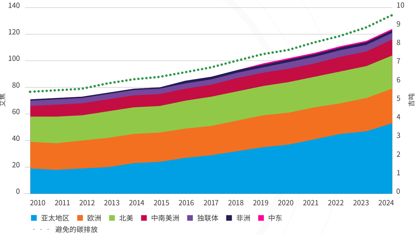
替代的碳排放和化石燃料使用量 (按区域划分)
