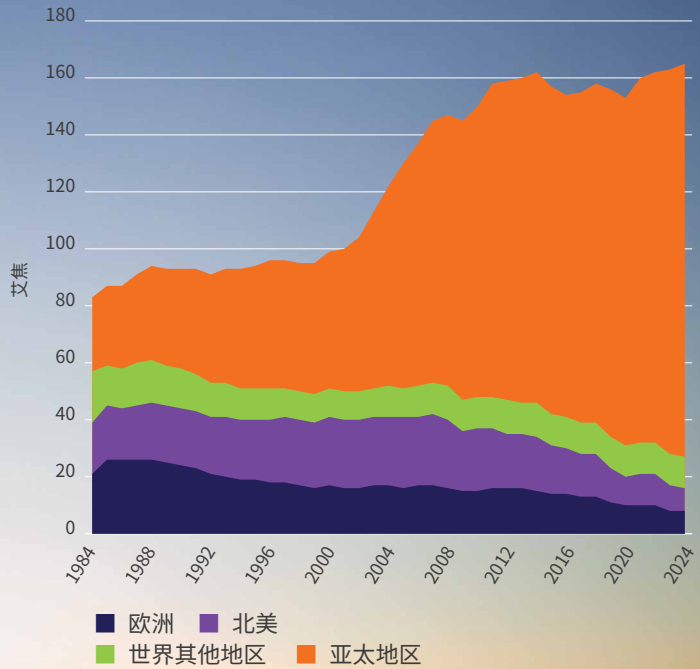
全球煤炭消耗量
