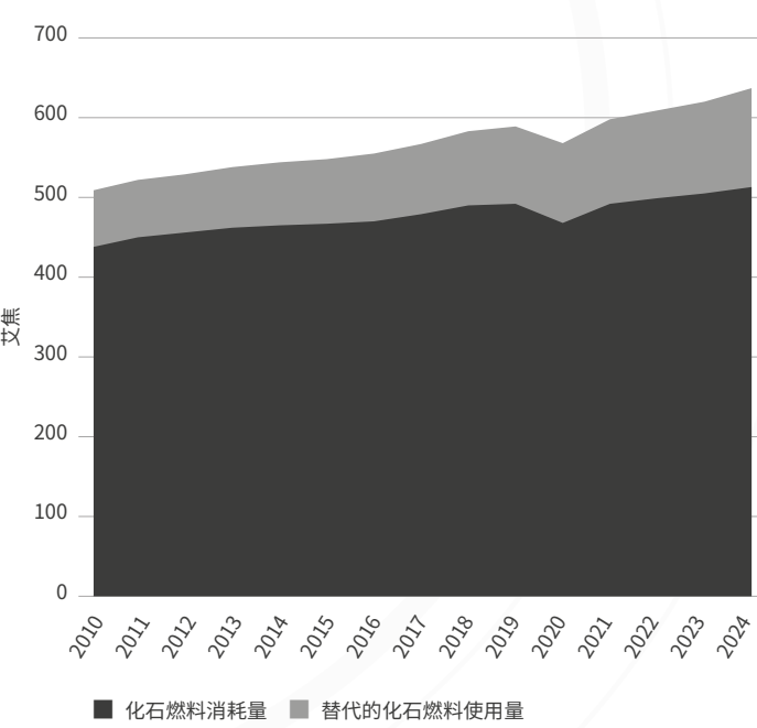
可再生能源和核能替代的化石燃料使用量
