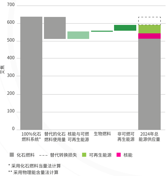
2024年, 可再生能源和核能助力全球降低对化石燃料的依赖, 提高能源系统效率
