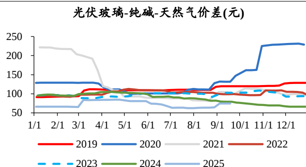
图52：当前光伏玻璃盈利能力低于2024年同期水平
