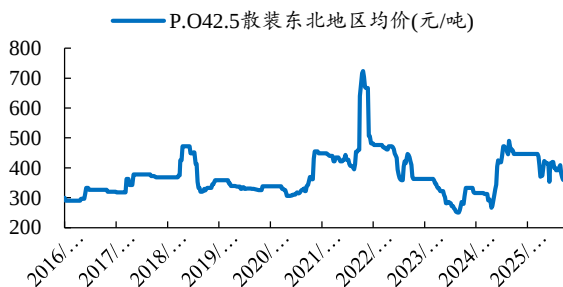
图10：本周东北地区水泥价格环比持平
