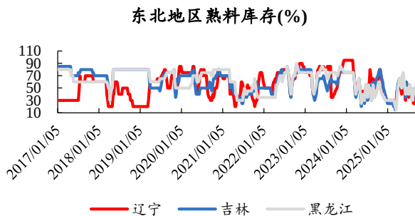
图11：本周东北地区熟料库存辽宁、黑龙江、吉林环比上涨
