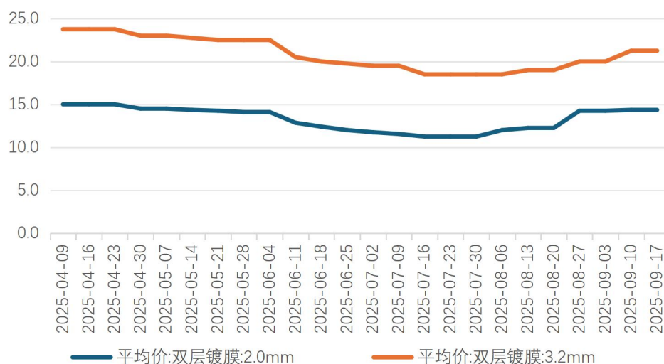
图表 18：光伏玻璃价格走势（元/平方米）
