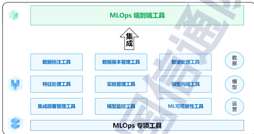
图 5 MLOps 工具分类一览
