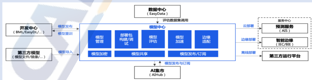
图 31 百度的模型管理流程图
