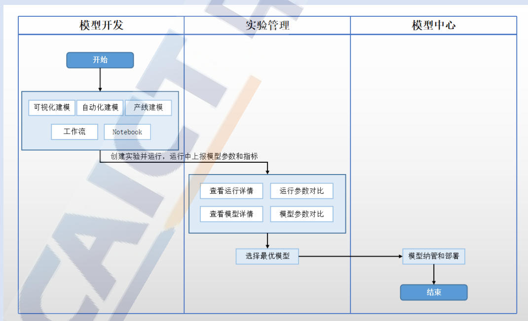
图 24 百度的实验管理流程图
