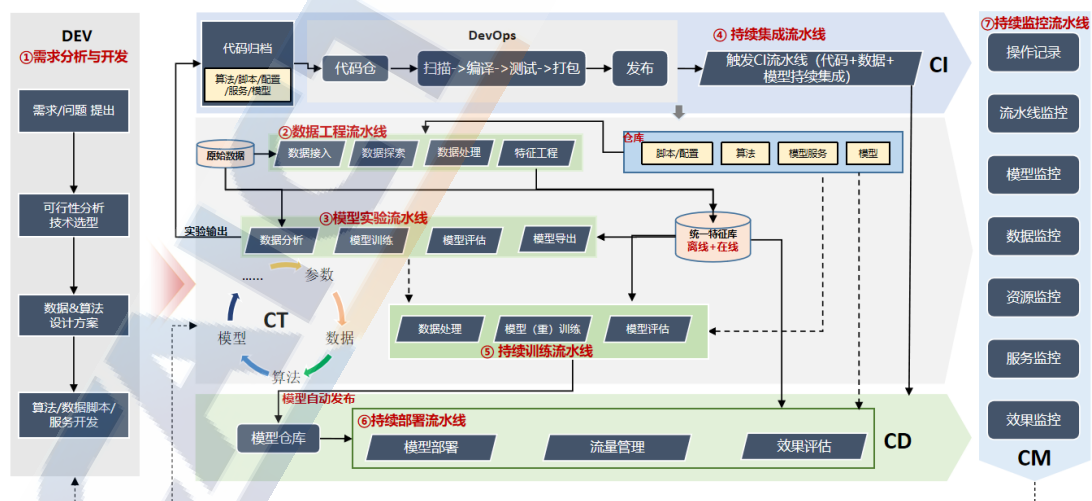
图 8 MLOps 流程架构示意图
