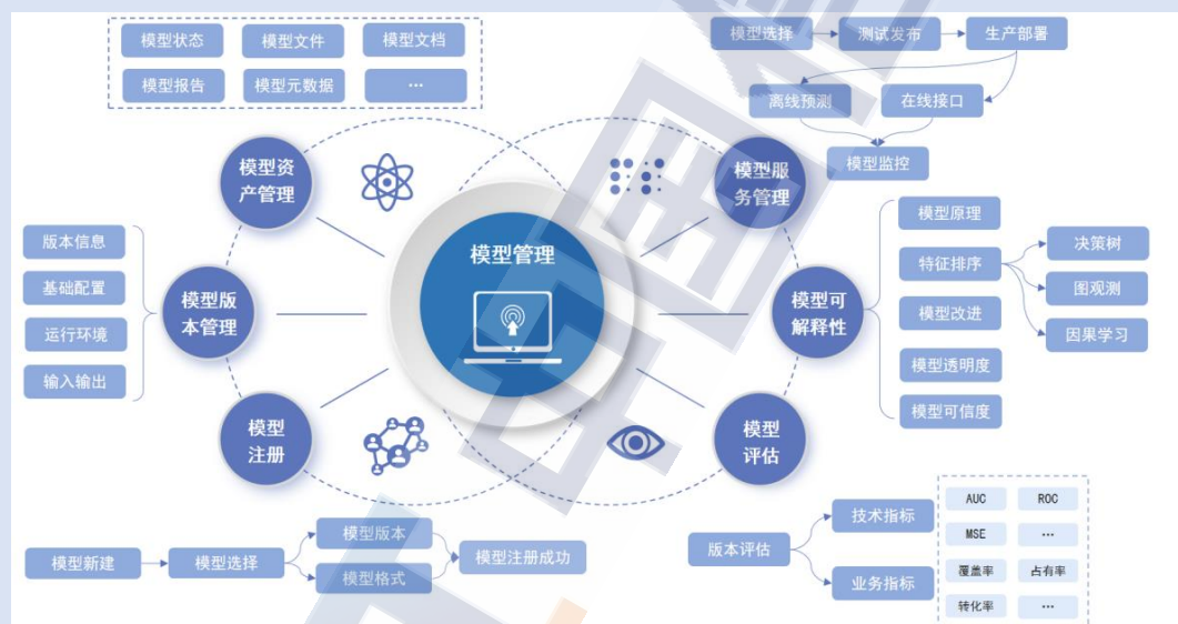
图 32 九章云极 DataCanvas 模型管理功能示意图
