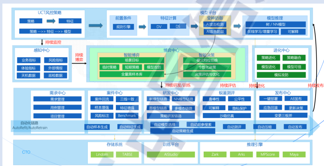
图 35 蚂蚁的 AntSecMLOps 架构图
