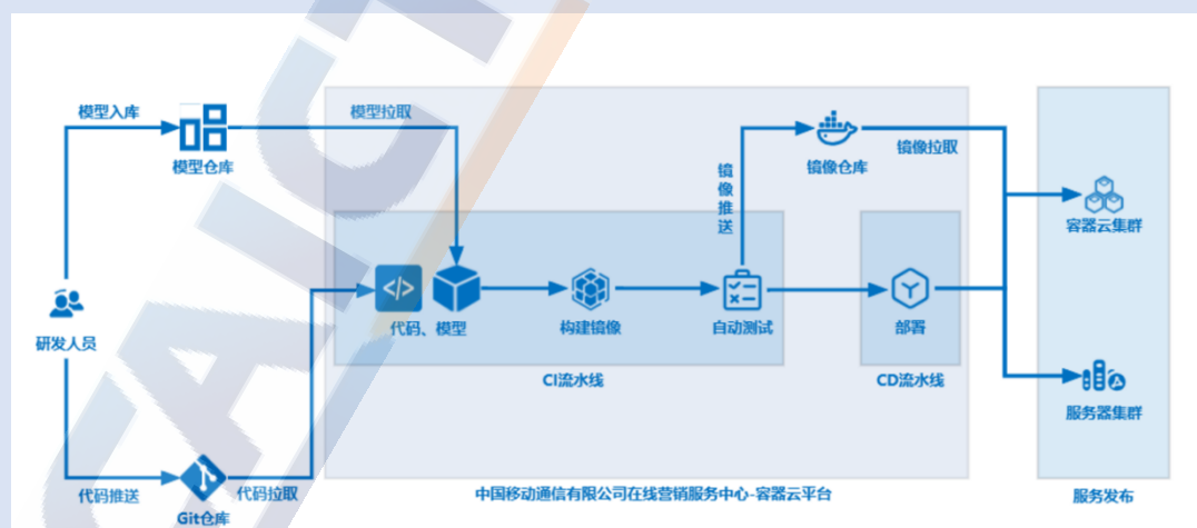
图 19 中移在线中心 Polaris MLOps 平台模型部署流程
