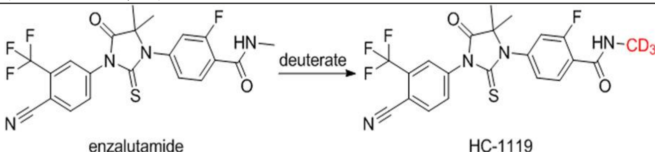
图表 1. HC-1119 化学结构
