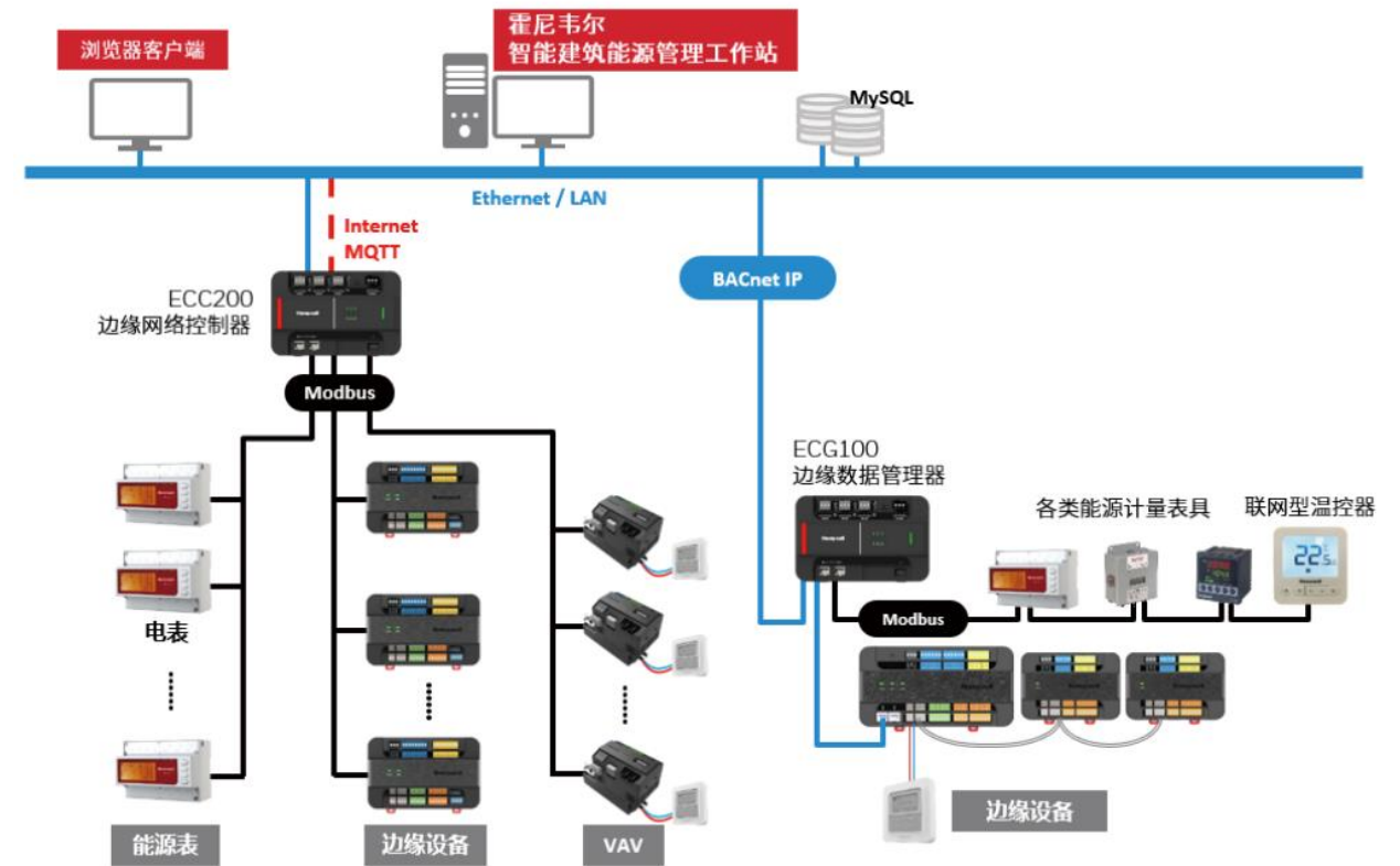
图 44：霍尼韦尔的系统架构
