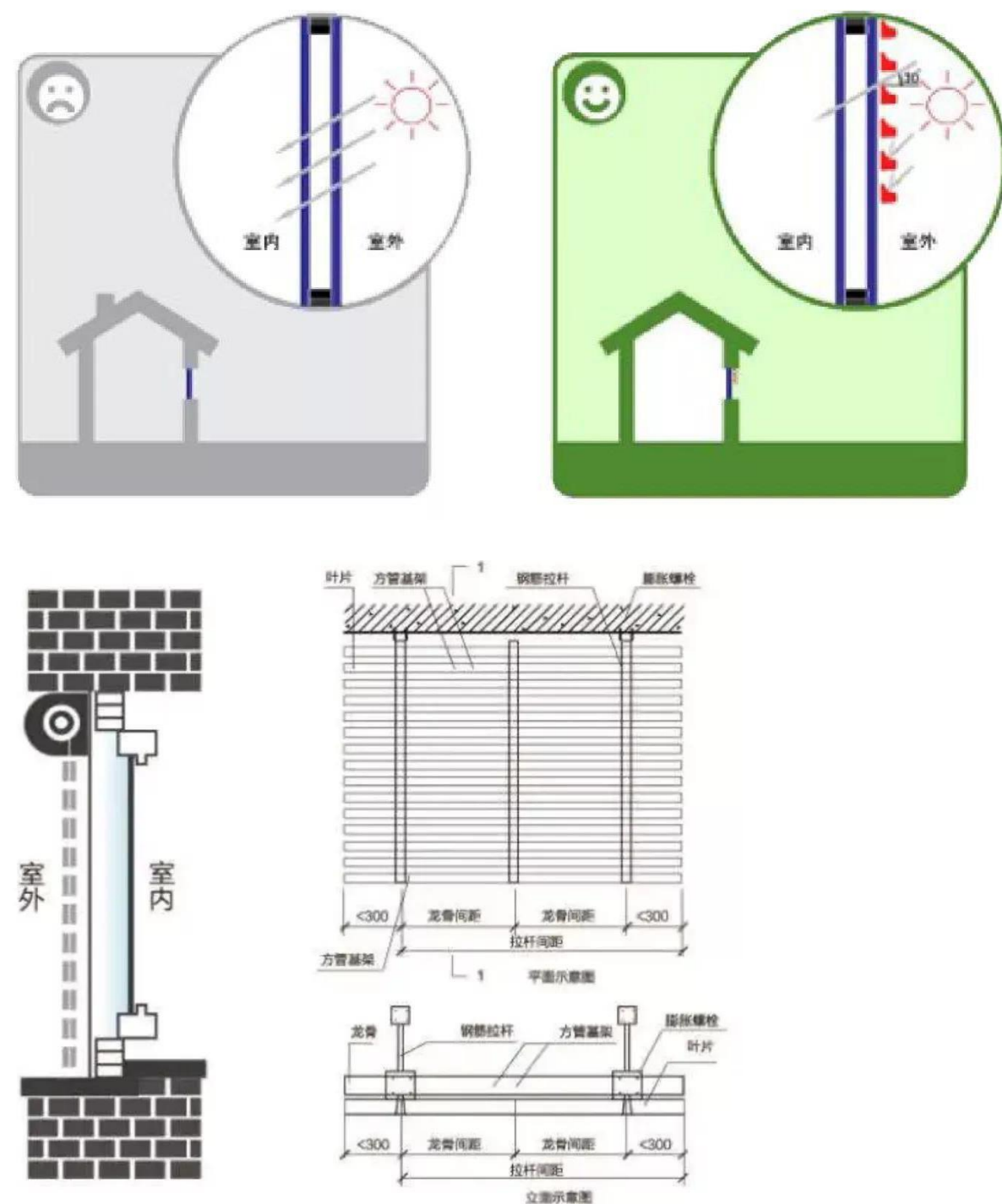
图 27：高效的外遮阳系统示意图
