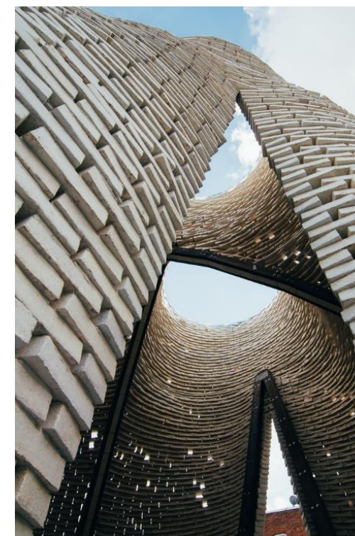
图 28: The Living 公司的 Hy-Fi 结构
