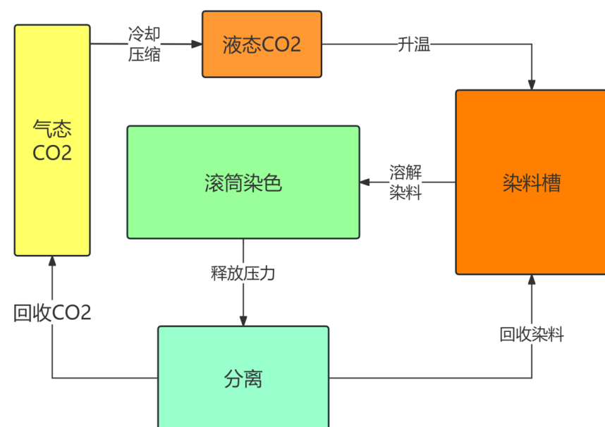
图 14：超临界二氧化碳流体染色流程
