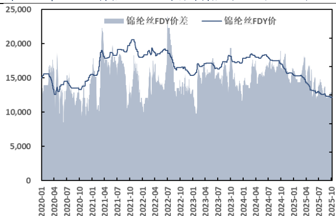
图 83: 锦纶 FDY 价格及 FDY 与切片价差 (元/吨, 元/吨)
