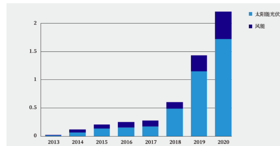
图 4.4 哈萨克斯坦太阳能和风能发电装机容量
