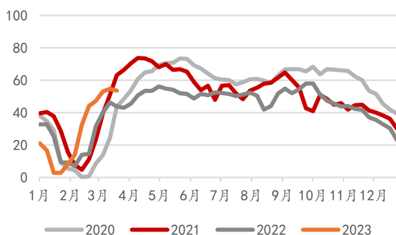
图表23: 全国水泥开工负荷(%)分年度变化
