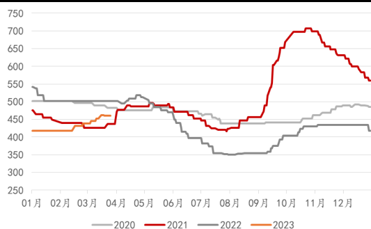
图表12: 华南水泥(P.O42.5散装)价格(元/吨)分年度
