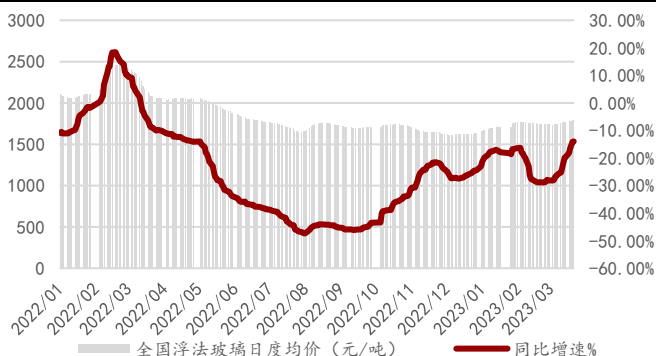
图表26: 5mm白玻价格分年度变化(元/吨)
