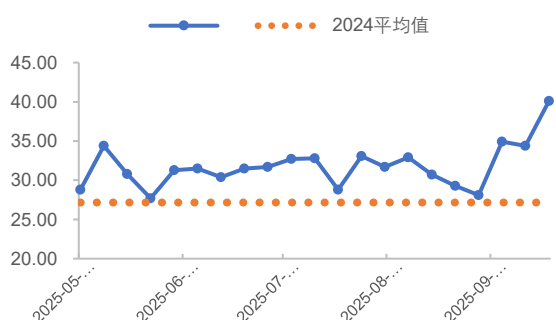
图7 石油沥青装置开工率 (%)
