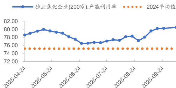
图24 焦化产能利用率 (%)
