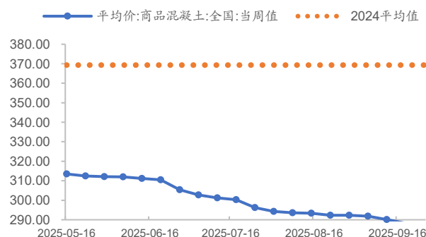
图38 混凝土价格（元/立方米）
