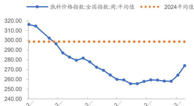
图36 熟料价格（元/吨）
