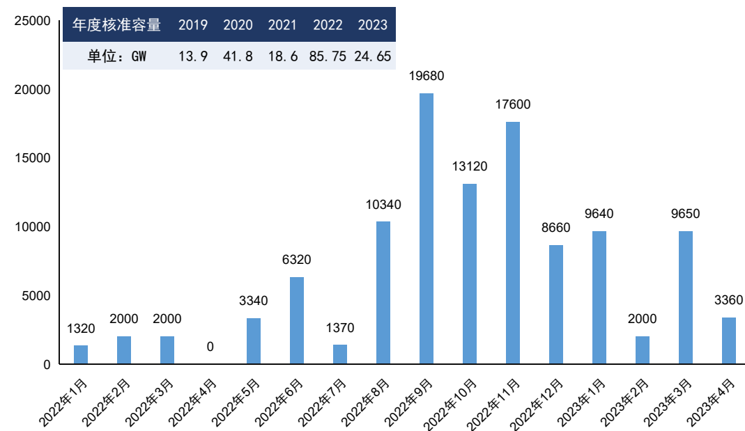
图35：煤电月度核准容量（MW）
