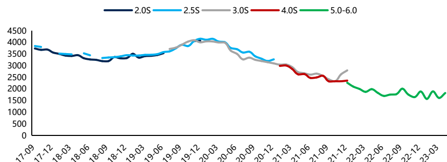
图16：陆上风机（不会附属设备）中标价格走势（含税，元/kW）
