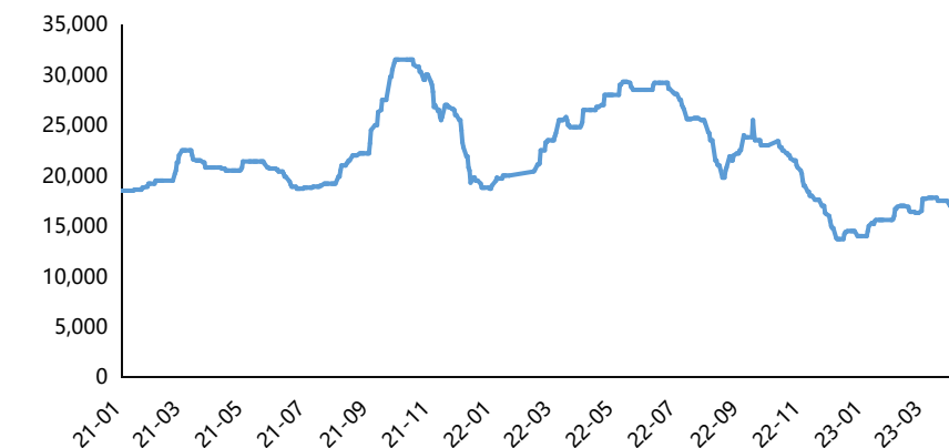
图30：线缆级EVA价格走势（元/吨）
