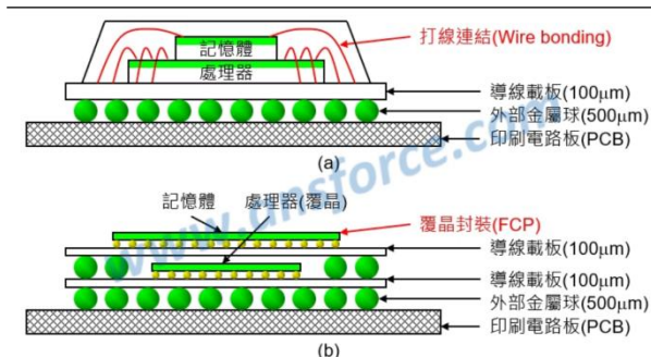
图13：FC（覆晶封装）与传统金线打线封装的区别示意
