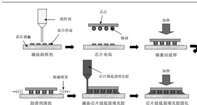
图14：FC 底填胶的使用流程
