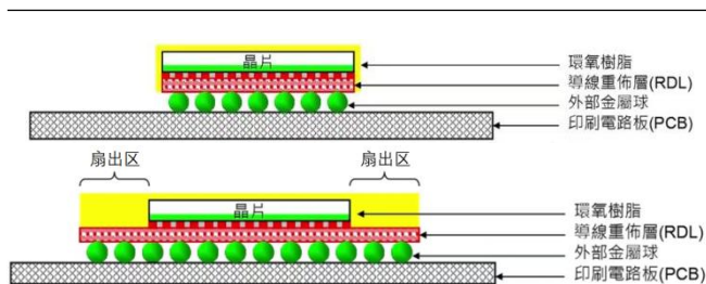
图12：扇入型封装与扇外型封装图示
