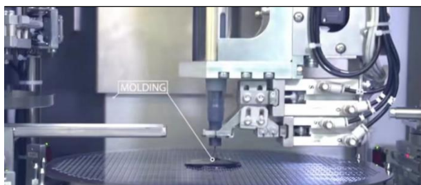
图11：LMC 在晶圆级封装中的实机演示
