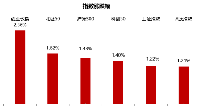
图2：指数涨跌幅（截至 2025/10/15）
