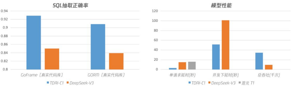
C1 基于真实代码库的SQL抽取能力优于通用大模型，模型性能全面占优
