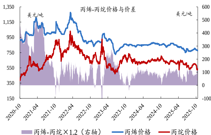
图23：本周丙烯-丙烷价差收窄
