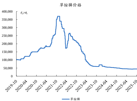
图52：本周草铵膦价格基本稳定
