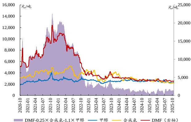
图39：本周 DMF 价差收窄
