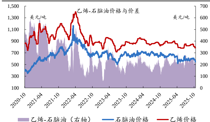
图19：本周乙烯-石脑油价差扩大
