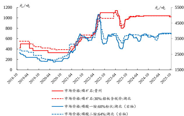
图14：本周磷矿石报价基本稳定
