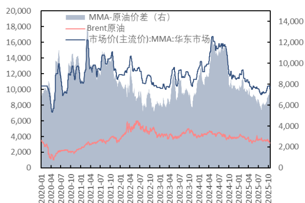
图 53: 原油、MMA 价格及价差 (元/吨, 元/吨)
