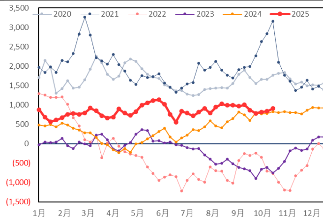
图 64: MEG 月度库存 (万吨)
