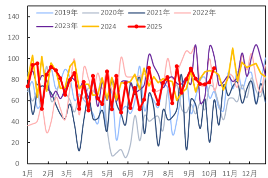
图 65：美国车用汽油净出口量（万桶/天）
