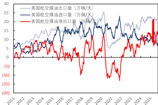
图 68：美国航空煤油进出口情况（万桶/天）
