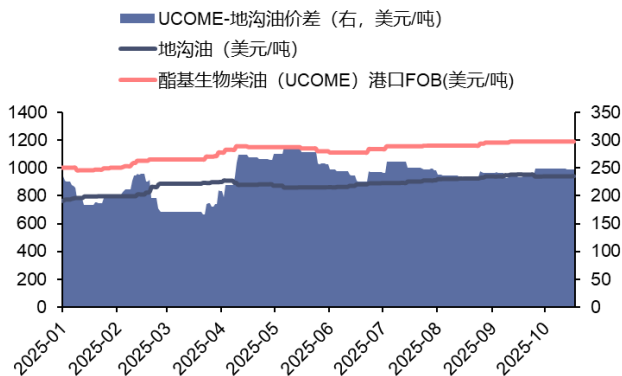
图 84：酯基生物柴油与地沟油价差（美元/吨，美元/吨）
