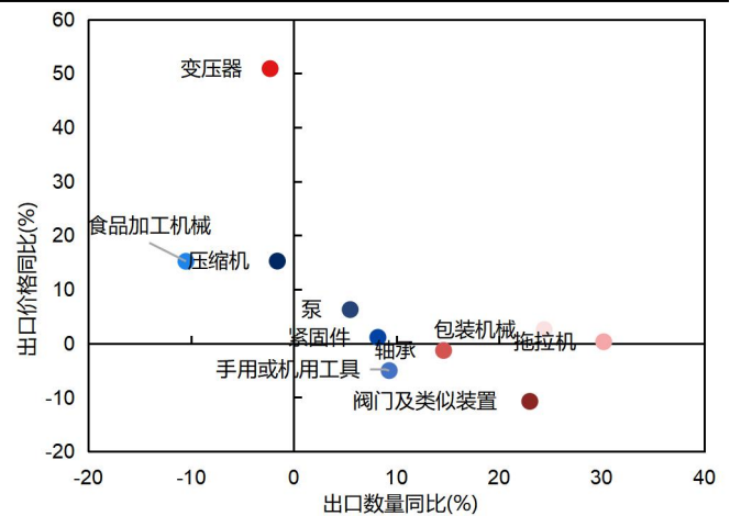
图表 19：9 月中国机械出口量价同比变化
