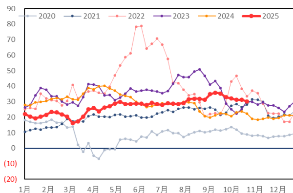
图 28: 原油、欧洲汽油价差 (美元/桶, 美元/桶)
