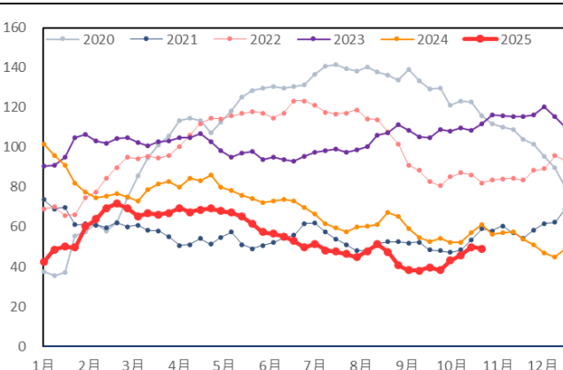
图 64: MEG 月度库存 (万吨)
