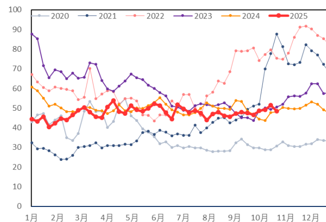
图 12：原油、国内航煤价差（美元/桶，美元/桶）
