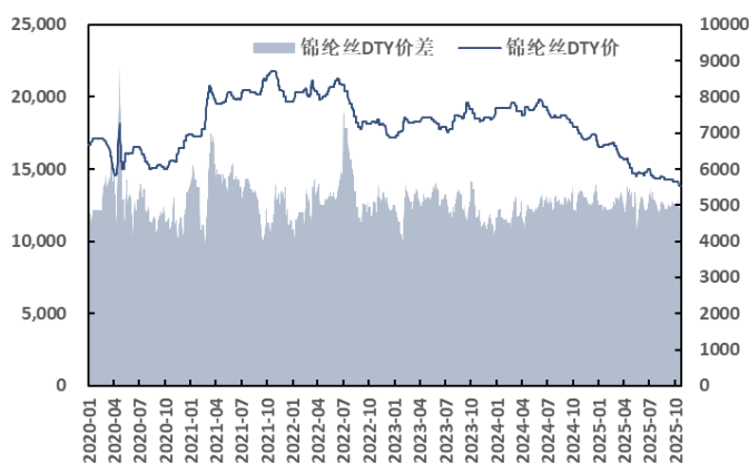
图 83: 锦纶 FDY 价格及 FDY 与切片价差 (元/吨, 元/吨)
