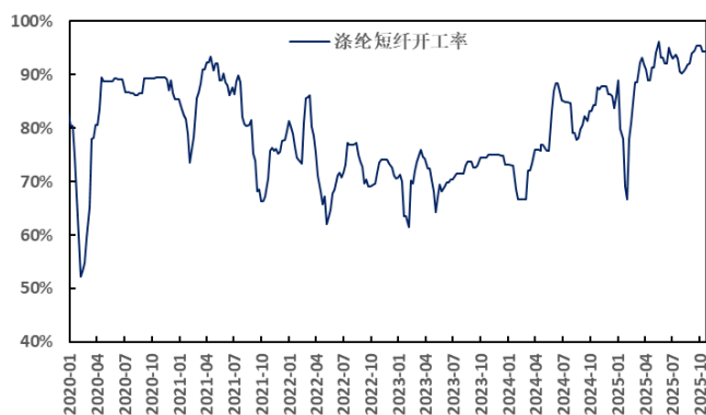
图 93: 2020-2025 年涤纶短纤开工率 (%)
