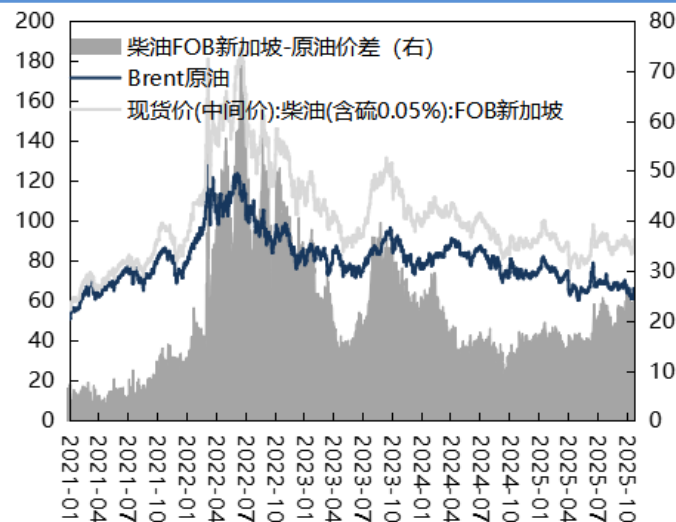
原油、新加坡柴油价格及价差（美元/桶，美元/桶）
