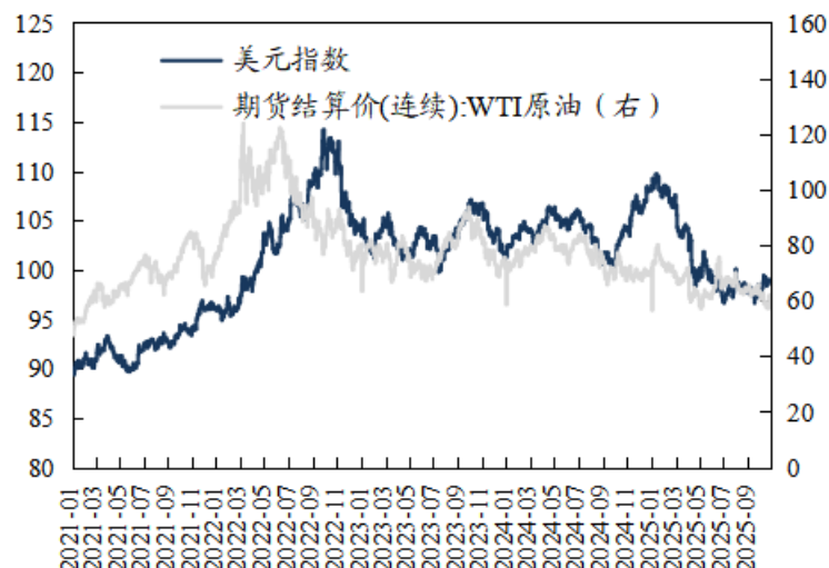
美元指数与WTI原油价格（点，美元/桶）
