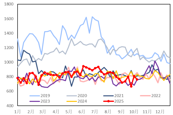
图 39: 美国东海岸 (PADD1) 商业原油库存 (万桶)
