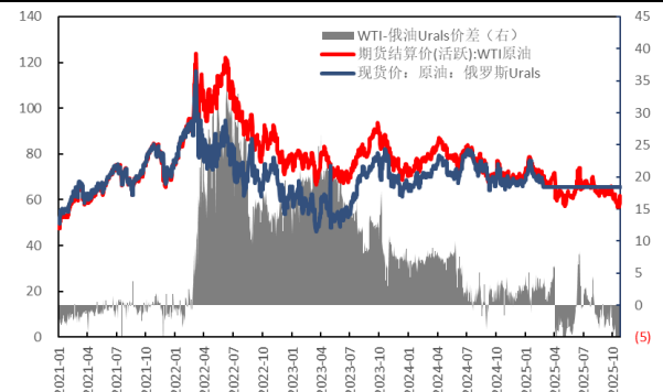
图 6: 布伦特、Urals 原油价格及价差 (美元/桶, 美元/桶) 图 7: WTI、Urals 原油价格及价差 (美元/桶, 美元/桶)
