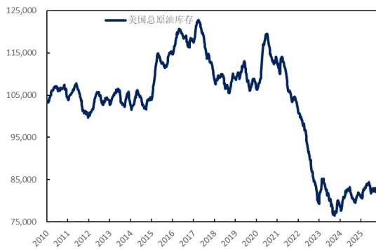
图 30：美国原油总库存（万桶）
