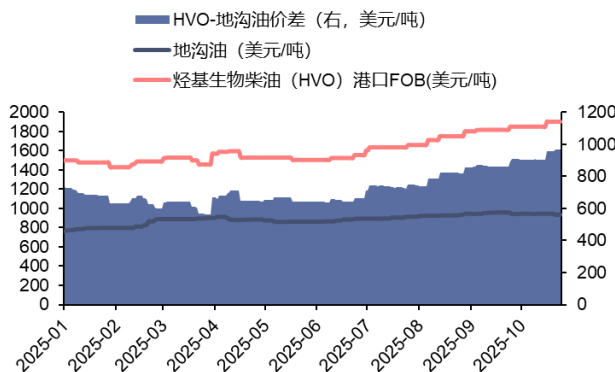
图 86：烃基生物柴油与地沟油价差（美元/吨，美元/吨）
