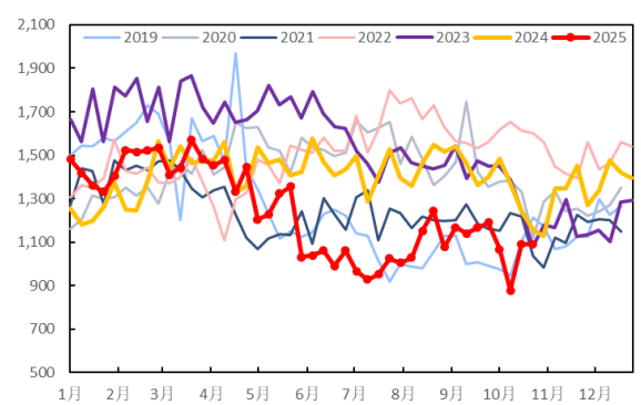
图 79: 新加坡汽油库存 (万桶)
