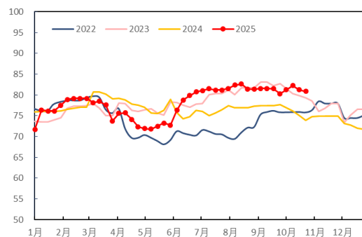
图 24: 中国主营炼厂开工率 (%)
