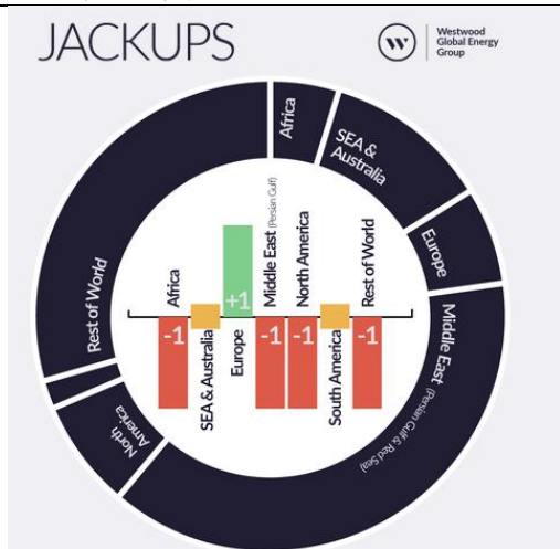
图 14：全球自升式钻井平台变化（座）
