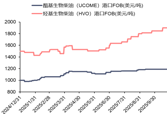
图 82：生物柴油港口 FOB 价格（美元/吨）
