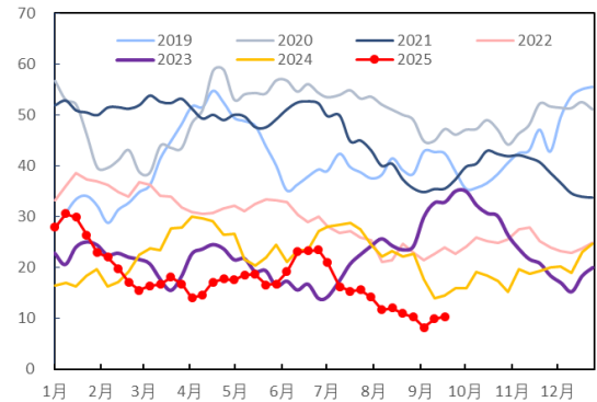
图 96：WTI 原油期货非商业净多头持仓量（万张）
