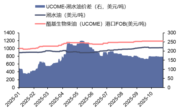
图 85：酯基生物柴油与泔水油价差（美元/吨，美元/吨）
