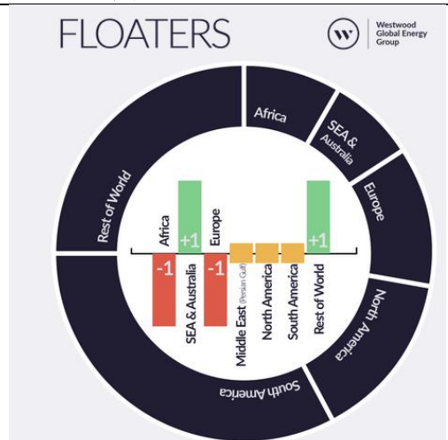
图 15：全球浮式钻井平台变化（座）
