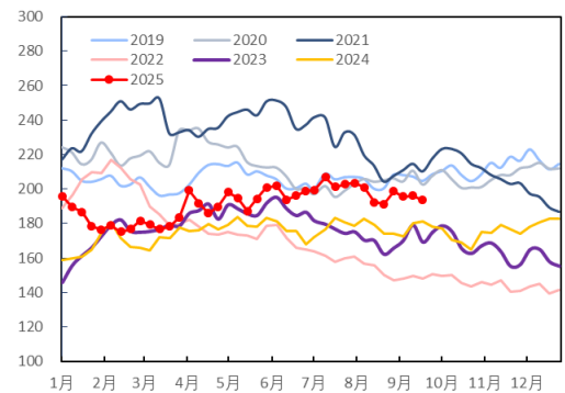
图 94：WTI 原油期货多头总持仓量（万张）
