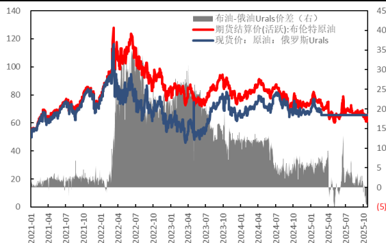
图 6: 布伦特、Urals 原油价格及价差 (美元/桶, 美元/桶) 图 7: WTI、Urals 原油价格及价差 (美元/桶, 美元/桶)
