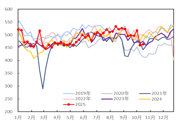
图 58：美国柴油产量（万桶/天）
