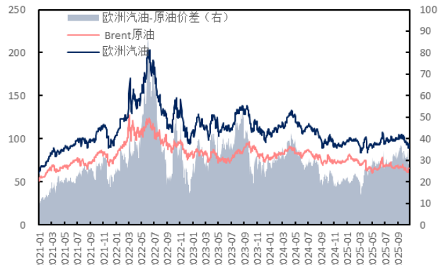
图 52：原油、欧洲汽油价格及价差（美元/桶，美元/桶）
