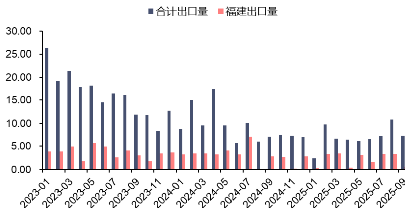
图 91: 酯基生物柴油月度出口量 (万吨)
