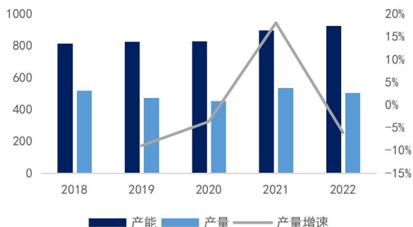
图45: 炭黑产能产量及增速 (万吨)
