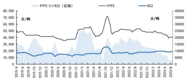
图26: PTFE 价格与价差跟踪
