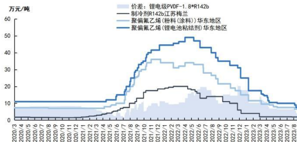
图27: PVDF 价格与价差跟踪
