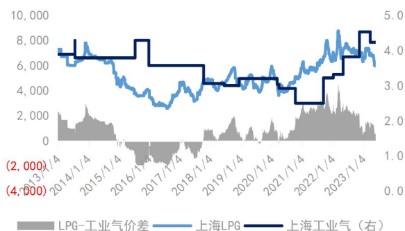
图16: 天然气（元/方）与 LPG（元/吨）经济性对比
