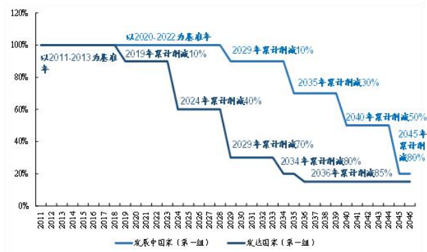
图19：发展中国家及发达国家三代制冷剂淘汰时间表
