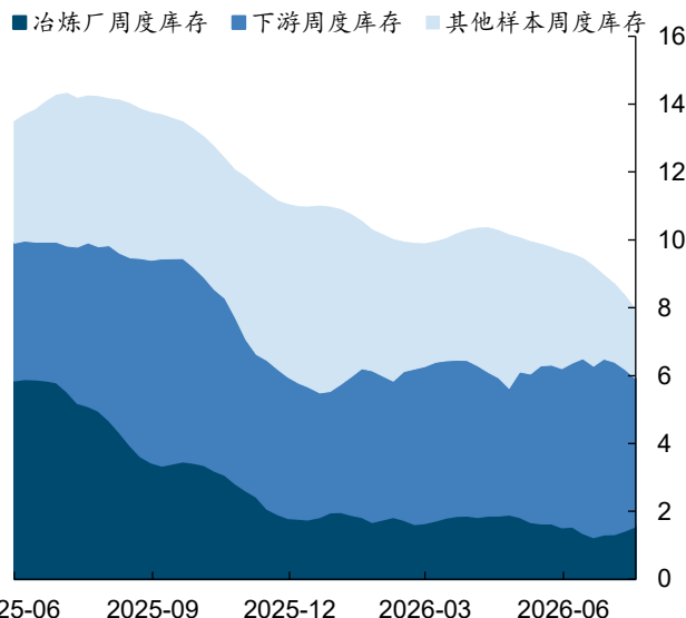
图表33：国内各环节碳酸锂库存（万吨）
